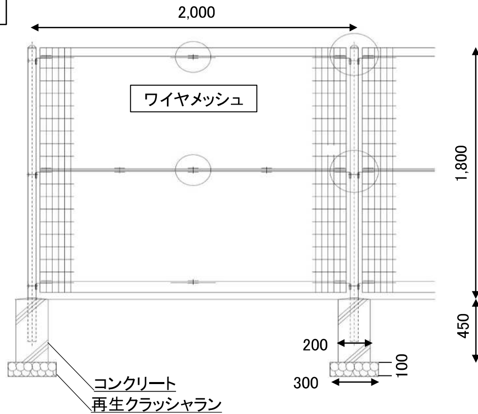
フェンス
