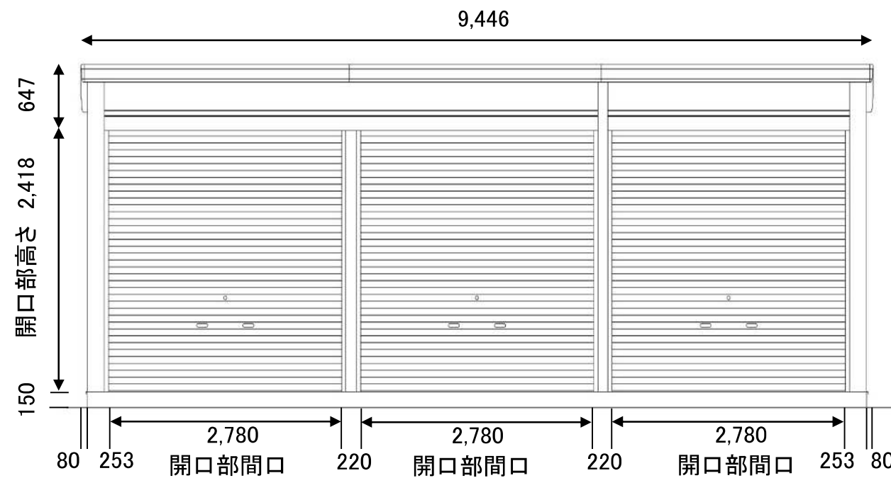
正面図
