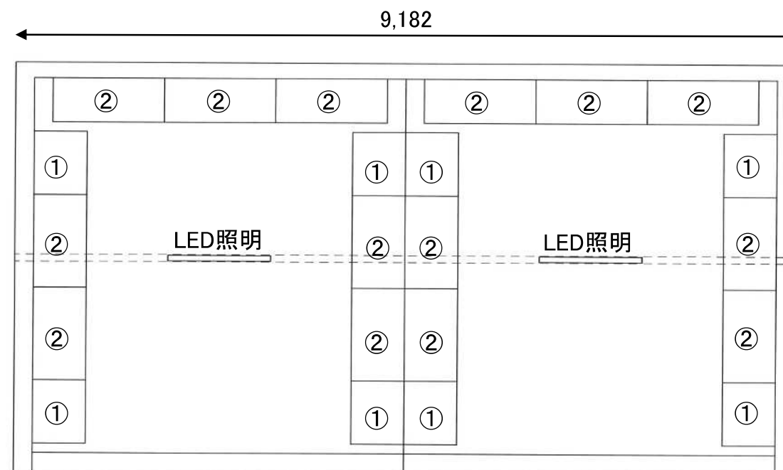
防災倉庫レイアウト(2分割)53.57㎡×1棟
