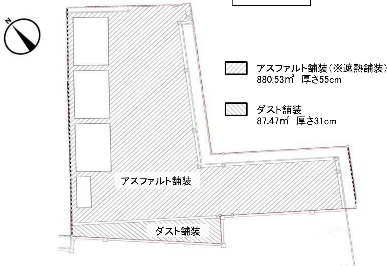
舗装平面図
