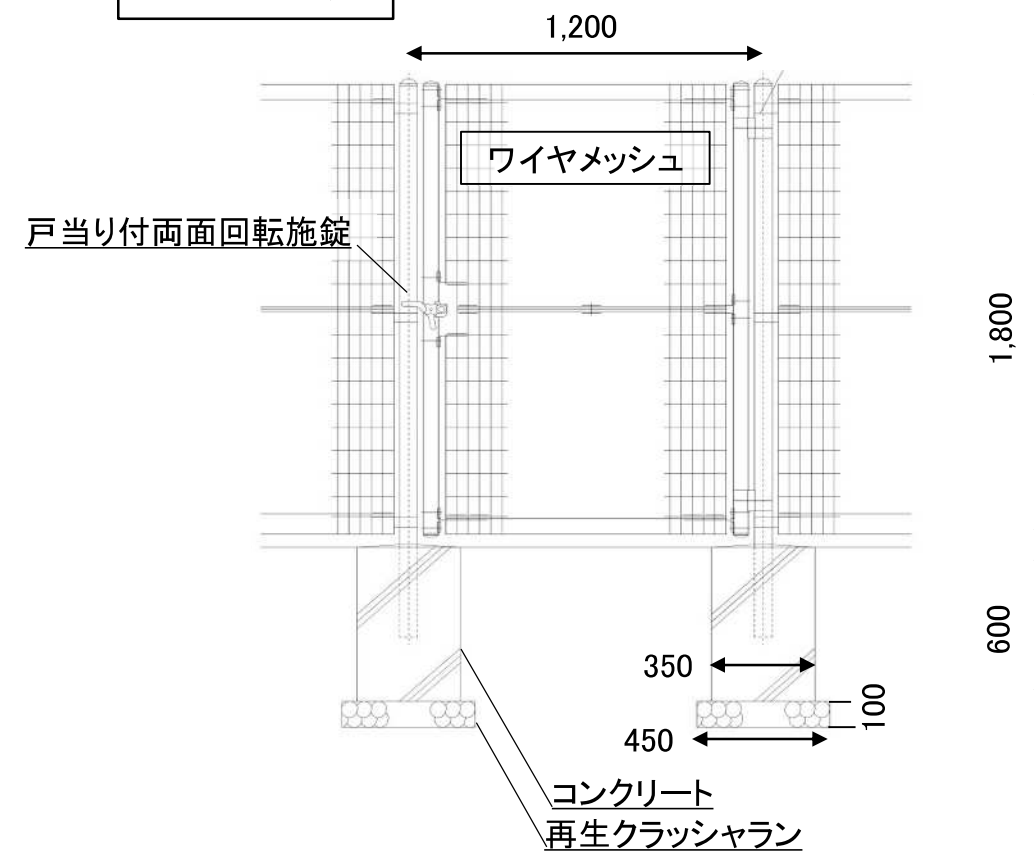
片開き門扉
