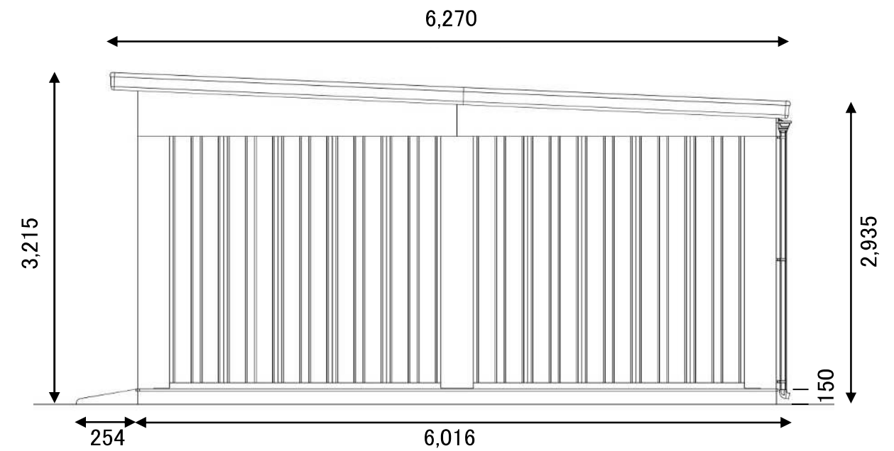
側面図
