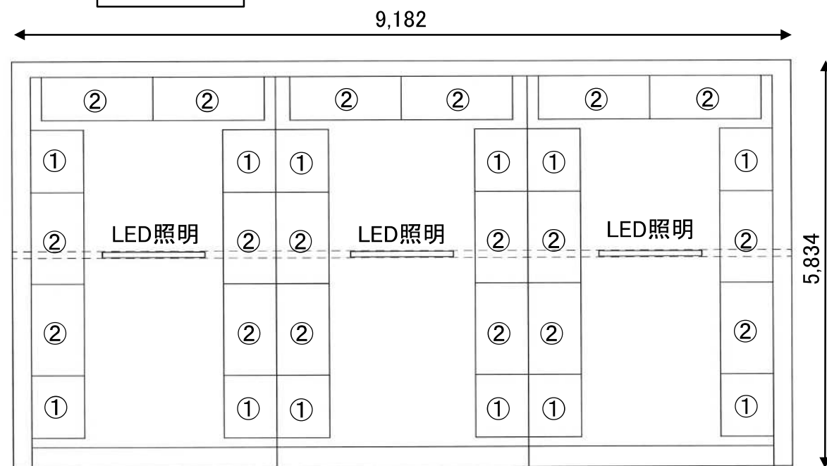
防災倉庫レイアウト(3分割)53.57㎡×2棟
